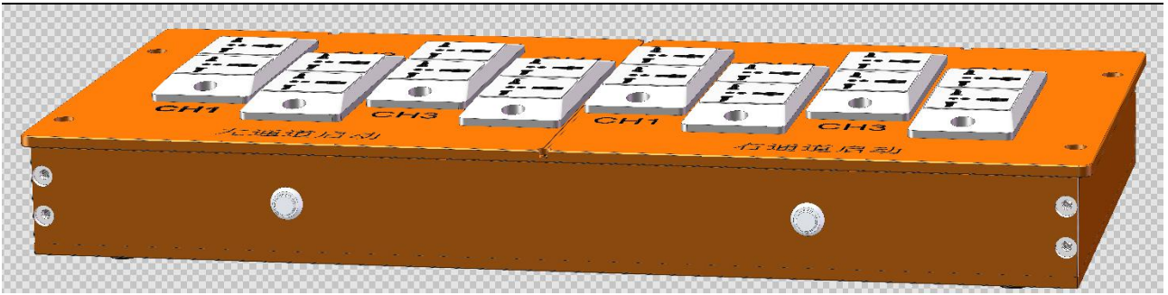
图 2.3.1 主机后面板
