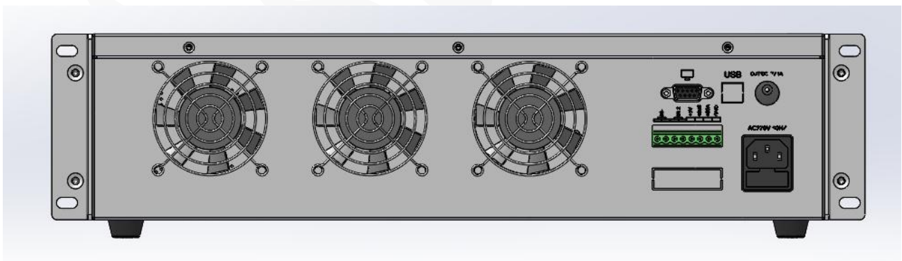
图 2.3.1 负载后面板
